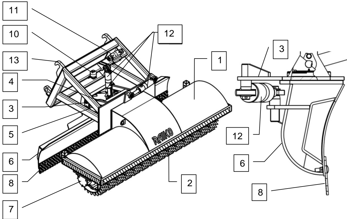
Kuva 7. Polannemurtaja P16 varaosakuvat
