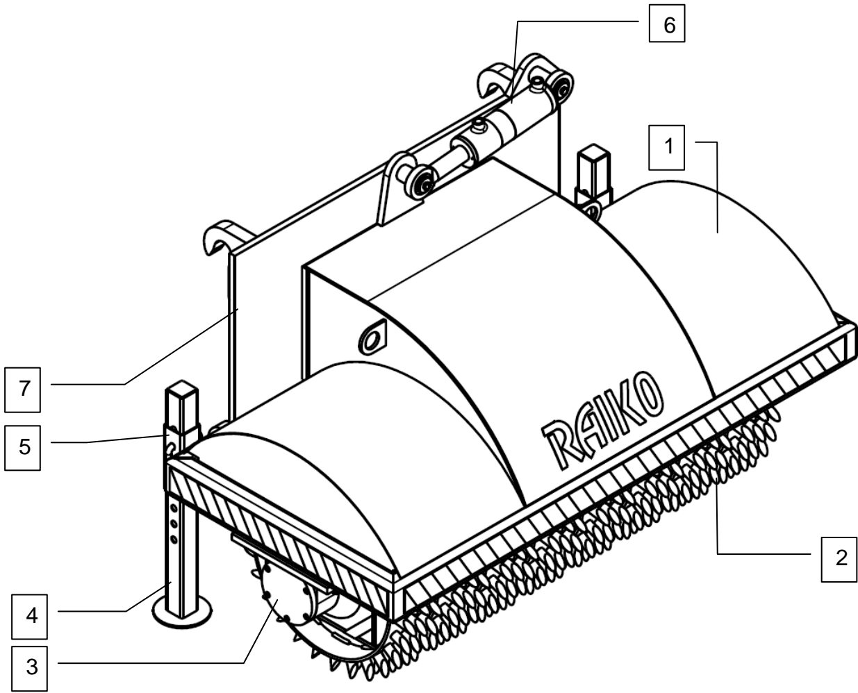
Kuva 5. Polannemurtaja T14-mallin varaosakuva
