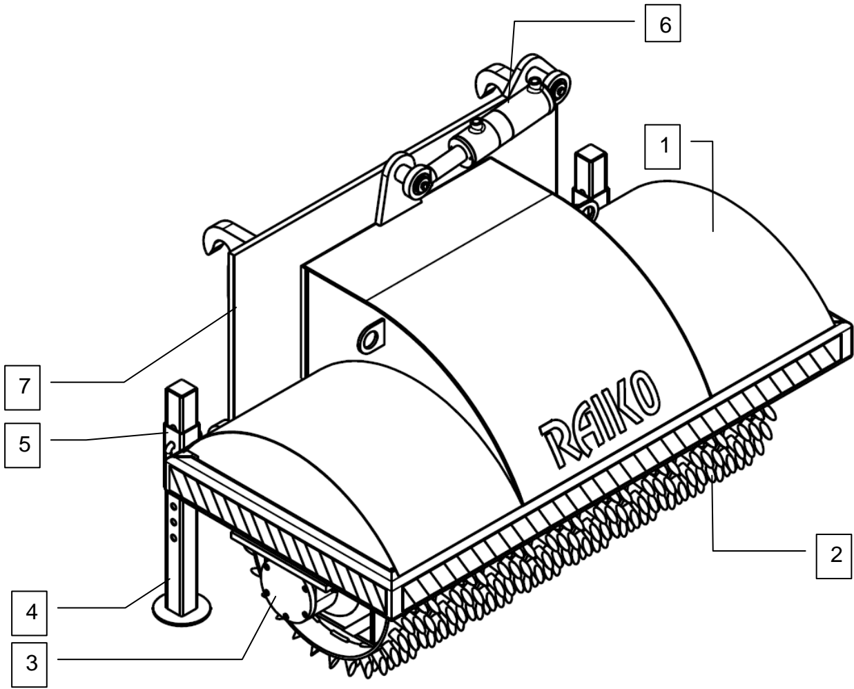
Kuva 5. Polannemurtaja T16-mallin varaosakuva
